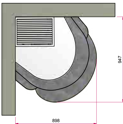
Изображение сверху М 1:20
